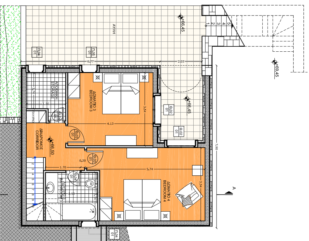
ΚΑΤΟΥΗ ΥΠΟΓΕΙΟΥ BASEMENT
