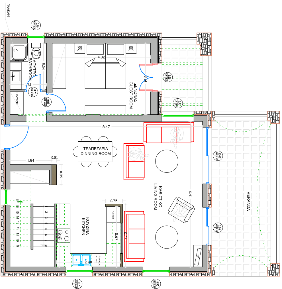
ΚΑΤΩΦΗ ΙΣΟΓΕΙΟΥ GROUND FLOOR
