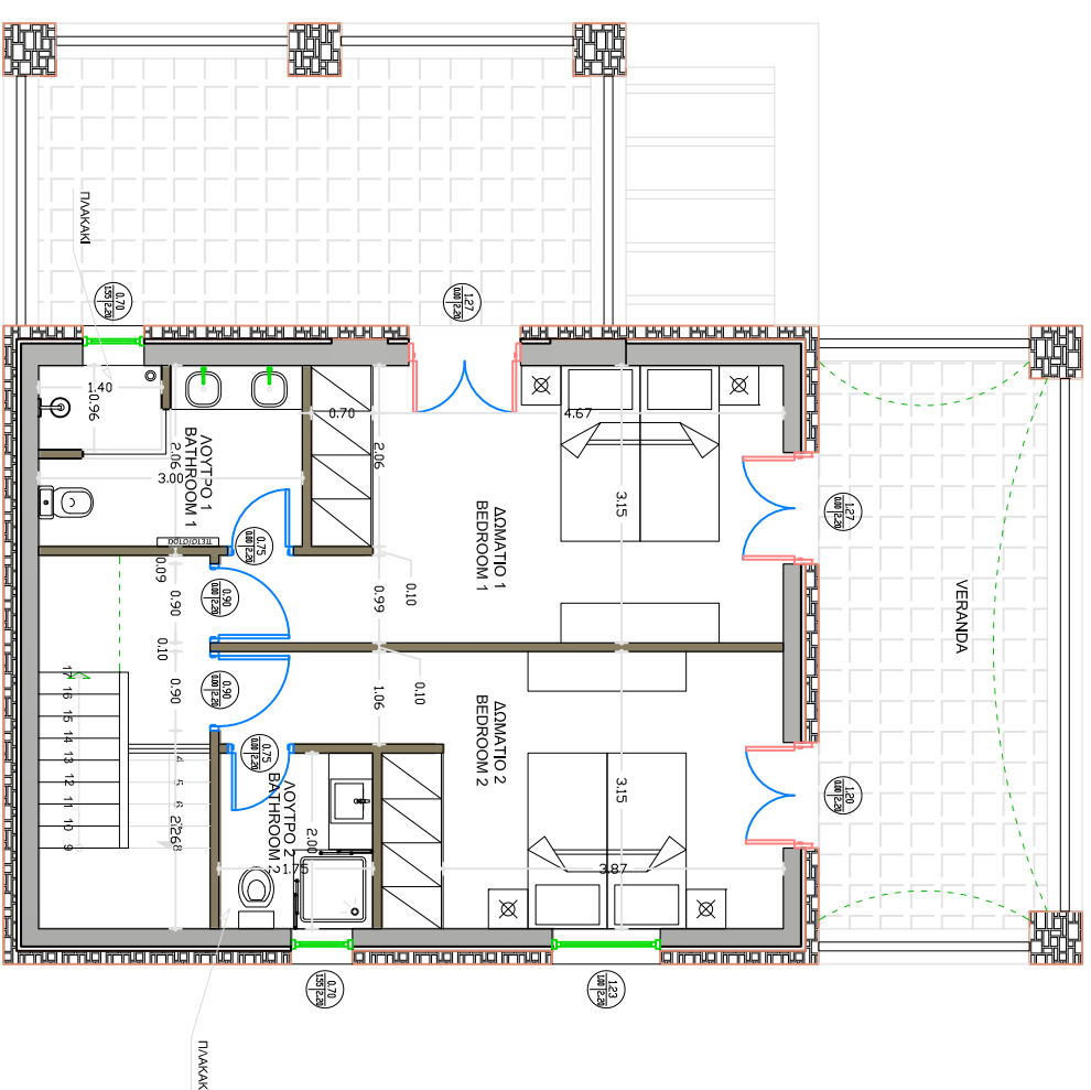
ΚΑΤΩΦΗ ΟΡΟΦΟΥ UPPER FLOOR
